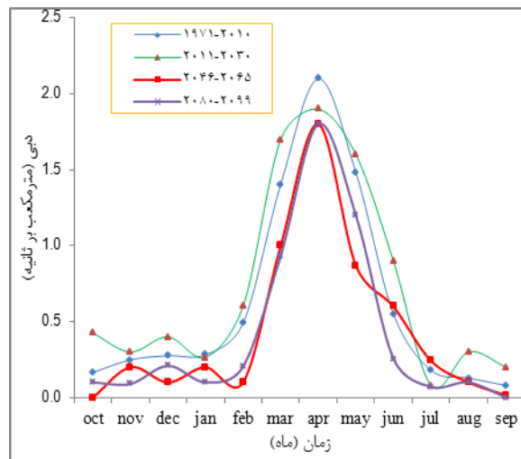
شکل ۵- هیدروگراف برآوردی حوزه بار طی دوره‌های مورد پیش‌بینی و تحت سناریو A1B, A2 و B1
